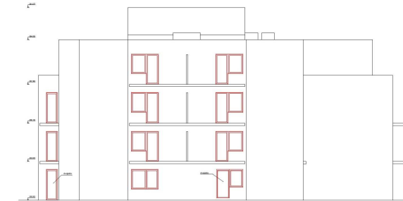
POHLED JIŽNÍ
